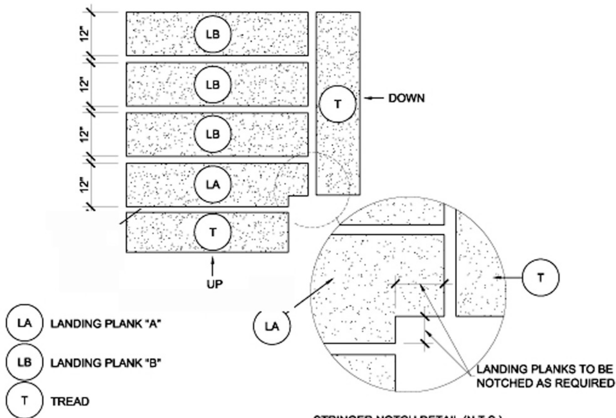
STRINGER NOTCH DETAIL (N.T.S.)
